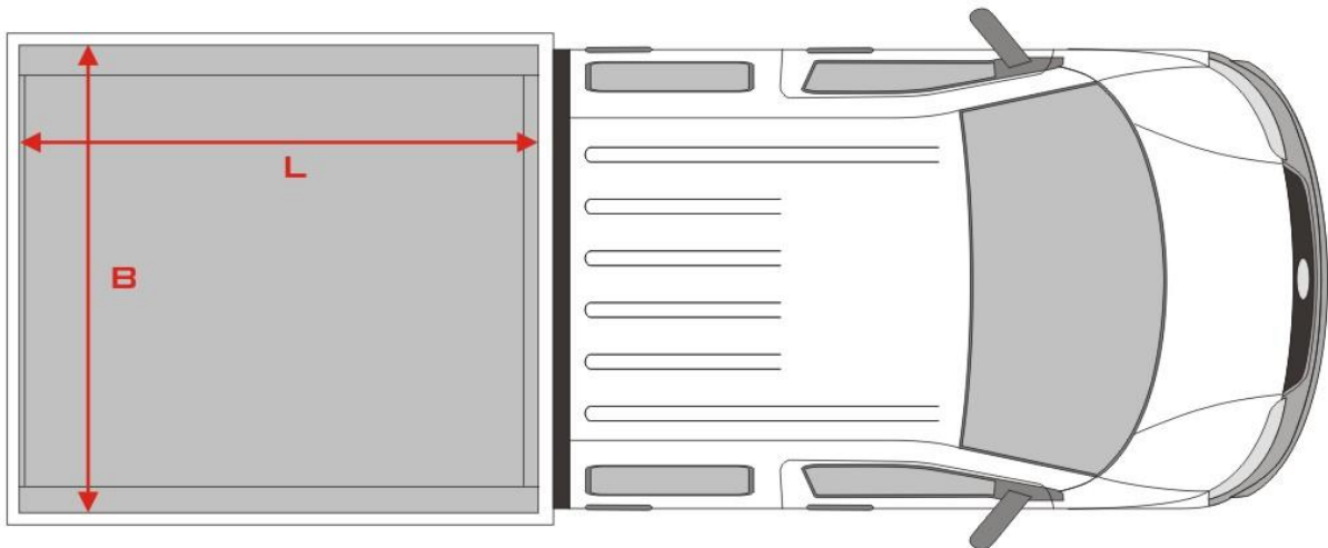
KASTENINNENMASS LÄNGE "L" x BREITE "B"
